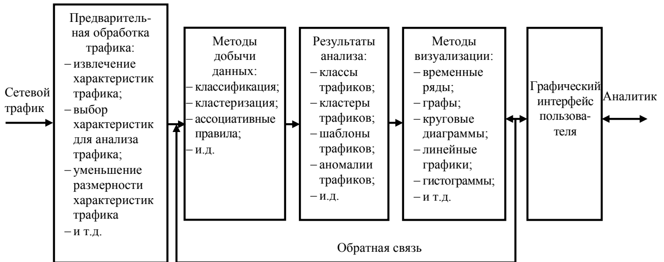
Рис.2. Модель визуализации мониторинга КС
