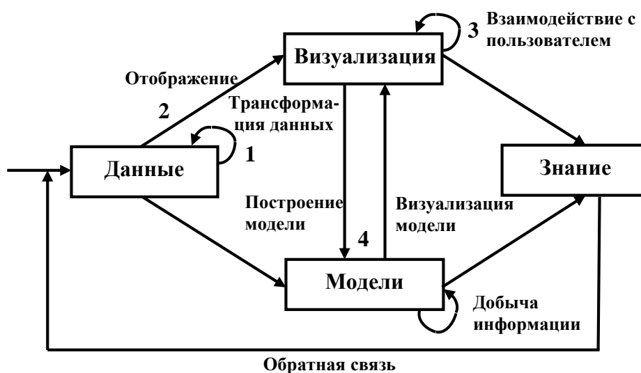
Рис.1. Процесс визуальной аналитики
